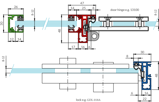
Office Basis-W Wall jamb
